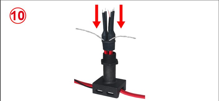
10：将绝缘套滑入发热电缆的导体，让接地导体留在外面。
